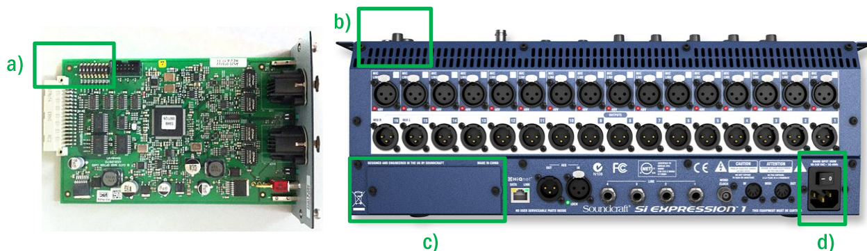
a)DIP switch b)Power On c)Slot Schede Opzionali d)Alimentazione
